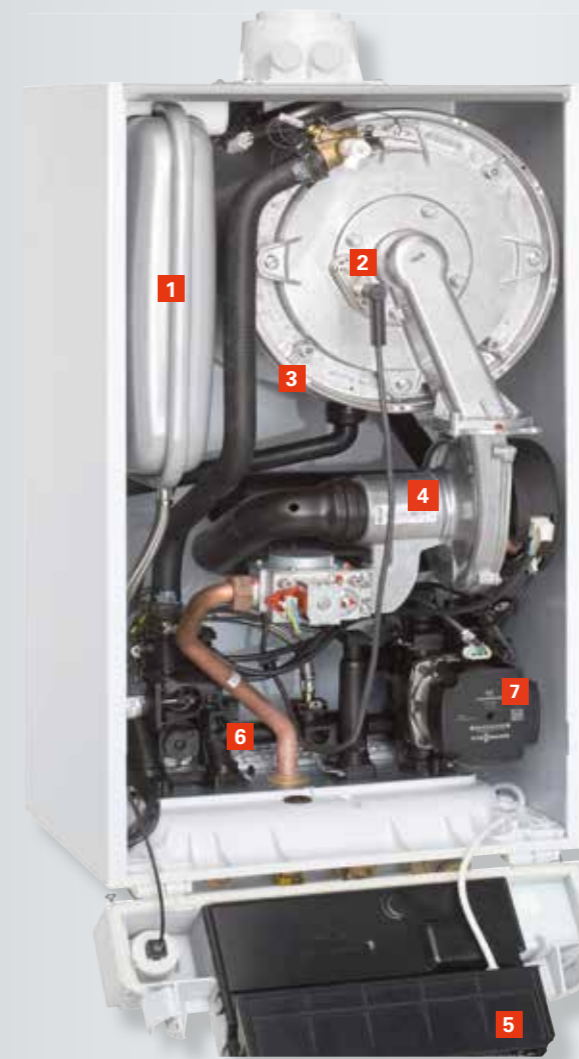
Caldera mixta con producción instantánea de A.C.S.
